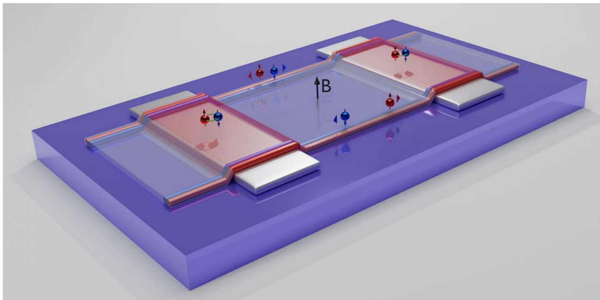
Schematische Darstellung des Versuchsaufbau: Zwischen zwei Kontakten (silber) befindet sich eine atomar dünne Schicht Wolframditellurid. Der Stromfluss in dem Material erfolgt nur an den Aussenkanten in sehr schmalen Kanälen. - Bild: Departement Physik, Universität Basel
